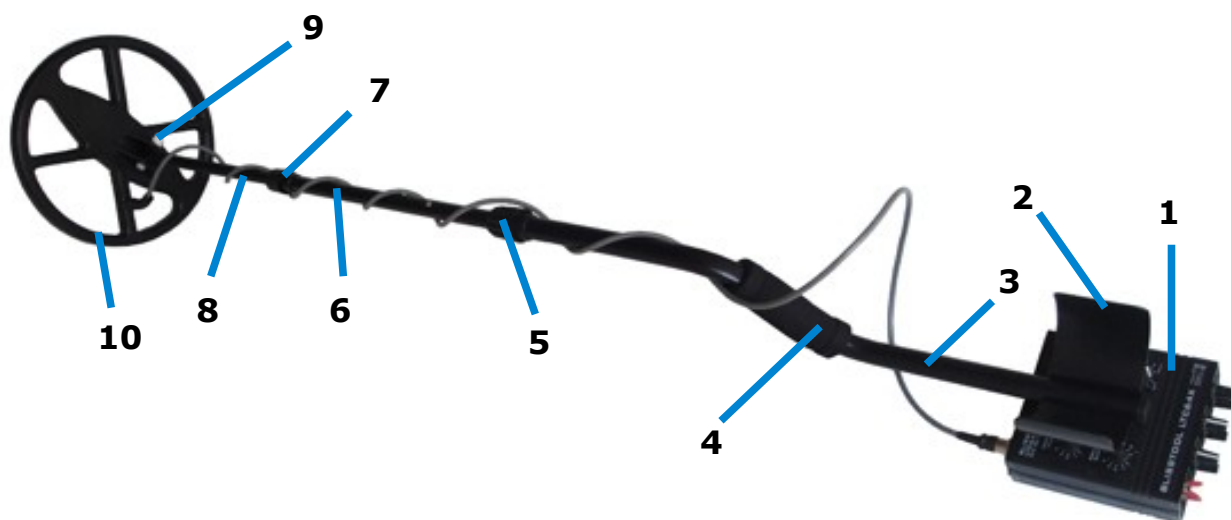
Рис.1 / Устройство металлоискателя BLISSTOOL LTC64X
