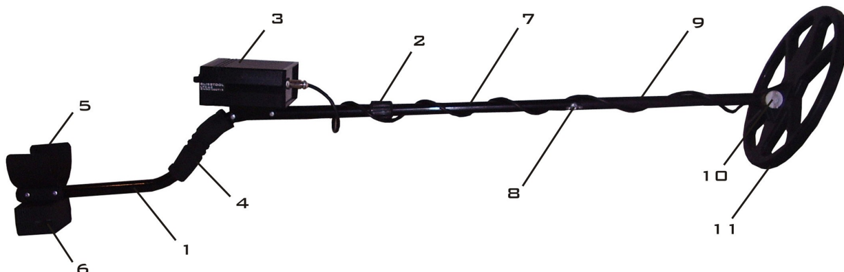
Фиг.1 / Устройство на металдетектор BLISSTOOL LTC42
